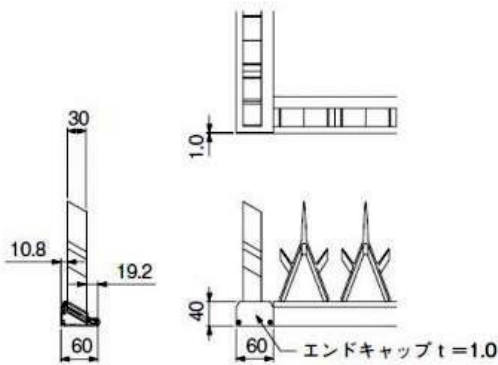
コーナー部納まり
